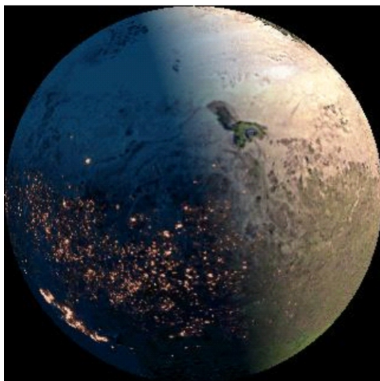
Gambar bumi yang difoto dari data satelit memperlihatkan sisi kanan pada siang hari dan sisi kiri pada malam hari (Sumber: http://www.fourmilab.ch/earthview/satellite.html )
